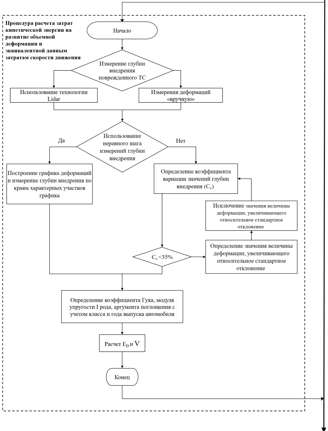
Рисунок 3.1 – Алгоритм проведения ДТЭ по разработанной методике оценки скорости движения автомобилей по их деформациям
