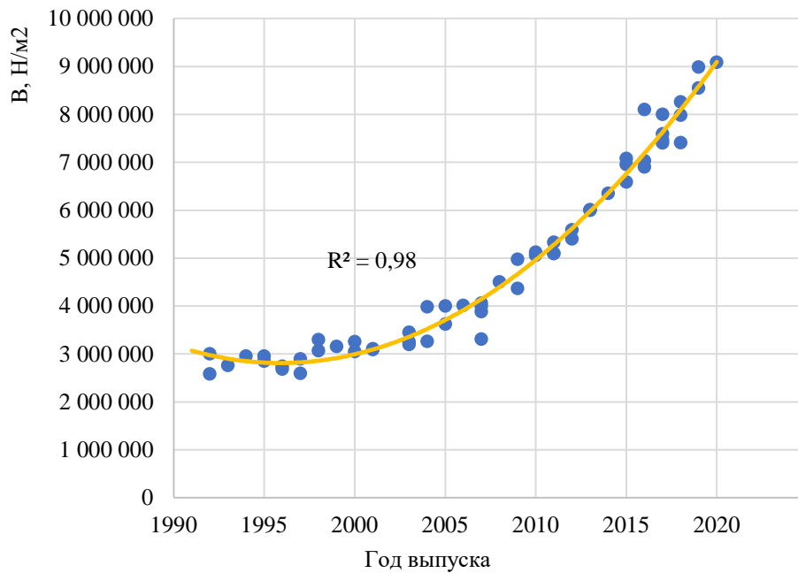
Рисунок П.Б.24 – Изменение значений модуля упругости I рода боковой части кузова автомобилей класса Small MPV в зависимости от года выпуска
