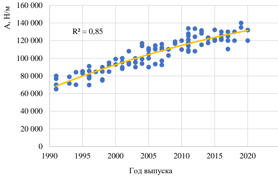
Рисунок П.Б.5 – Изменение значений коэффициента Гука фронтальной части кузова автомобилей класса Small family car в зависимости от года выпуска
