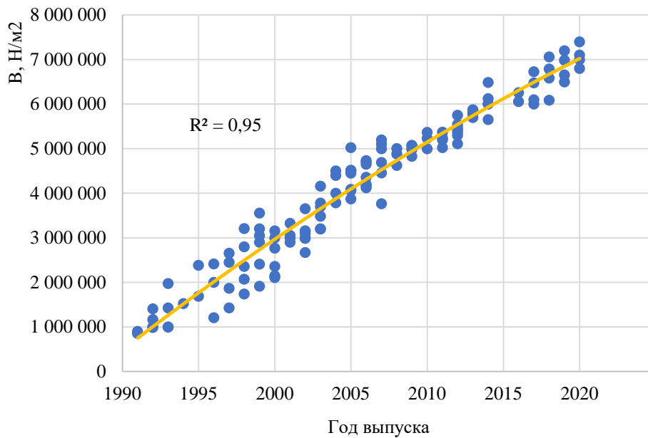
Рисунок П.Б.12 – Изменение значений модуля упругости I рода боковой части кузова автомобилей класса Large family car в зависимости от года выпуска
