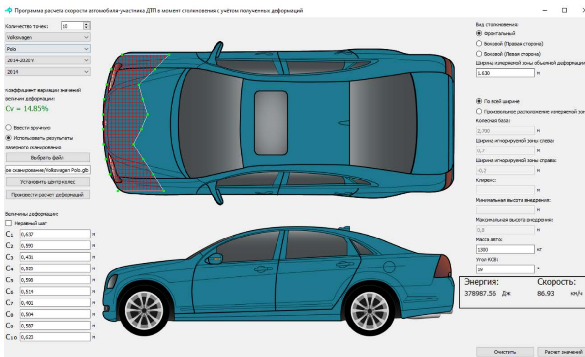
Рисунок 4.15 – Результат расчета затрат кинетической энергии и соответствующей данным затратам скорости автомобиля Volkswagen Polo
