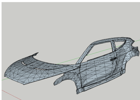
Рисунок 2.27 – 3D-модель кузовных элементов прямой контактной зоны а/м Hyundai Veloster, в деформированном состоянии (вид слева)
