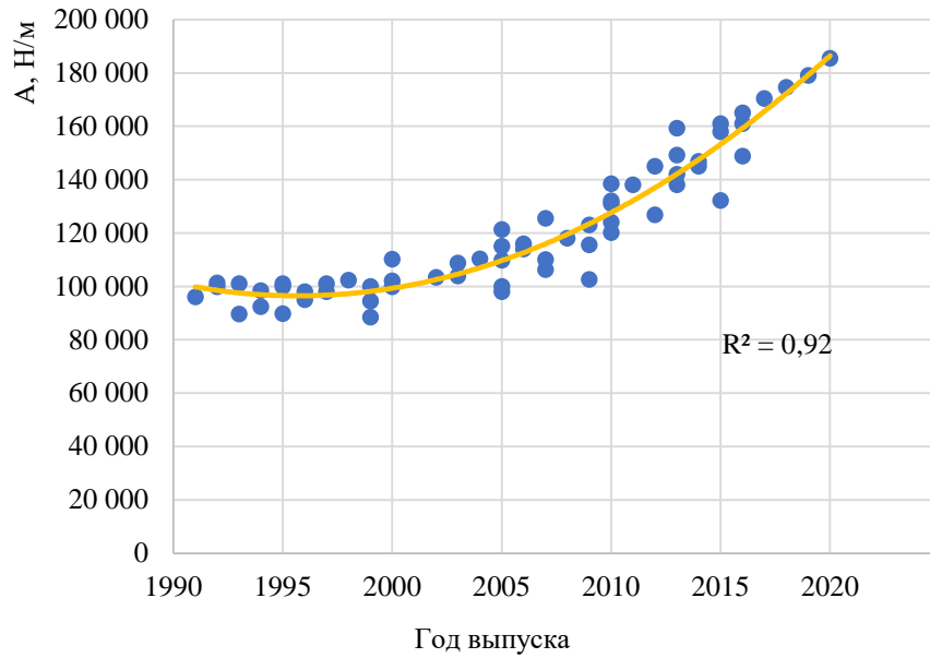
Рисунок П.Б.21 – Изменение значений коэффициента Гука фронтальной части кузова автомобилей класса Small MPV в зависимости от года выпуска
