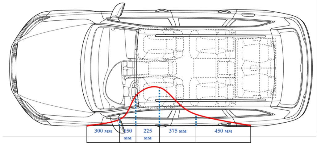
Рисунок 2.17 – Схема участков измерения глубин внедрения с неравным шагом
