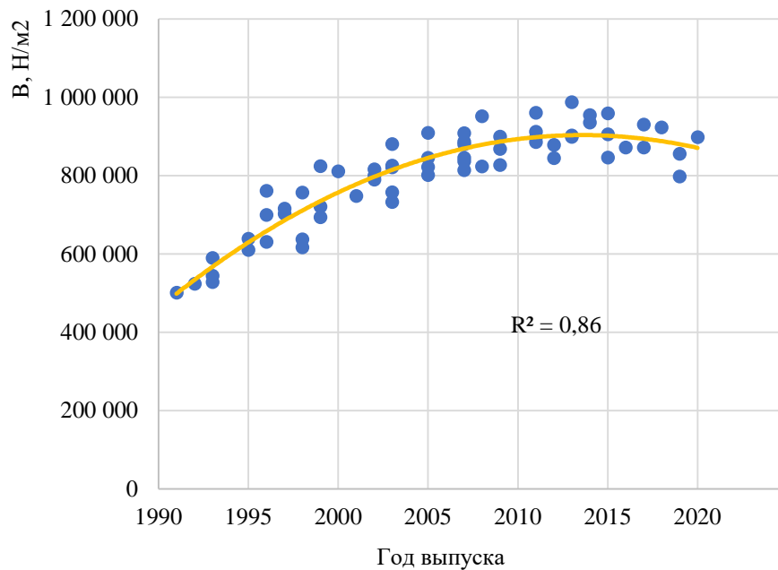
Рисунок Б.2.34 – Изменение значений модуля упругости I рода фронтальной части кузова автомобилей класса Large Off-Road 4×4 в зависимости от года выпуска
