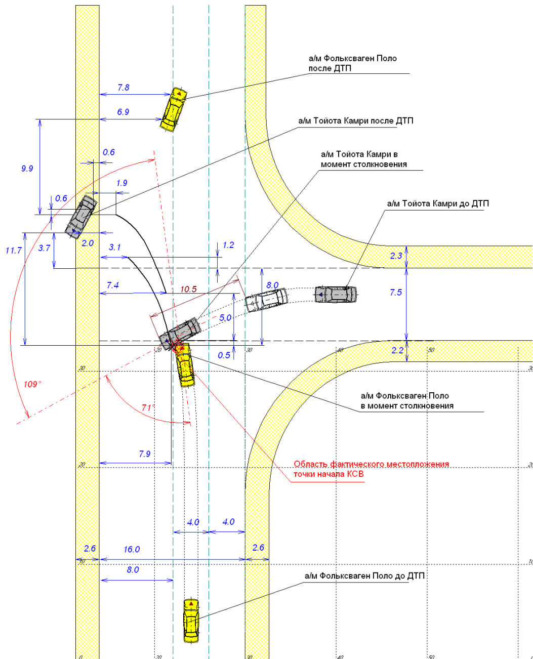
Рисунок 4.16 – Масштабная расчетная схема ДТП с участием автомобилей Volkswagen Polo и Toyota Camry
