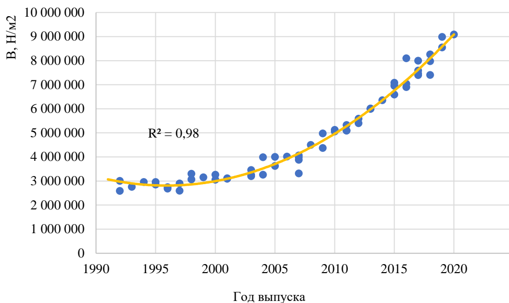
Рисунок 2.21 – Изменение значений модуля упругости I рода боковой части кузова автомобиля класса Small MPV в зависимости от года выпуска
