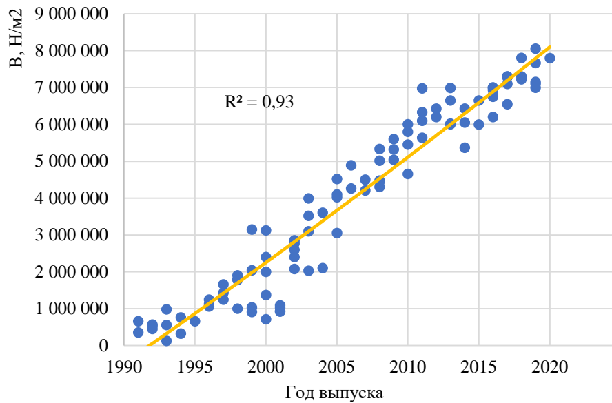
Рисунок П.Б.16 – Изменение значений модуля упругости I рода боковой части кузова автомобилей класса Executive car в зависимости от года выпуска
