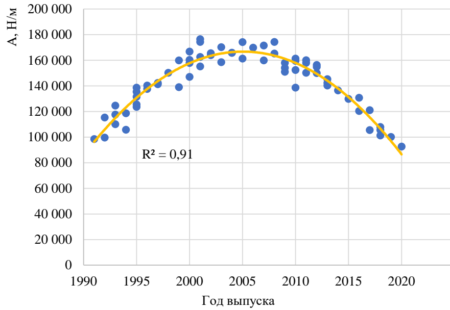
Рисунок П.Б.27 – Изменение значений коэффициента Гука боковой части кузова автомобилей класса Large MPV в зависимости от года выпуска
