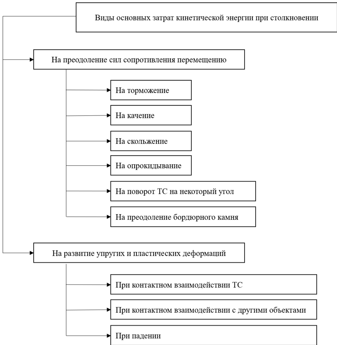
Рисунок 1.9 – Виды основных затрат кинетической энергии
