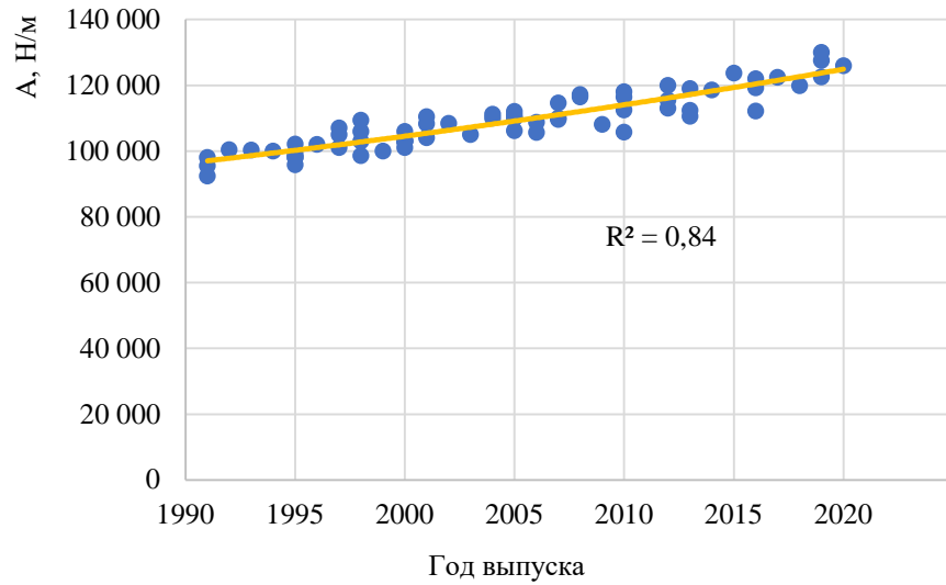
Рисунок П.Б.13 – Изменение значений коэффициента Гука фронтальной части кузова автомобилей класса Executive car в зависимости от года выпуска
