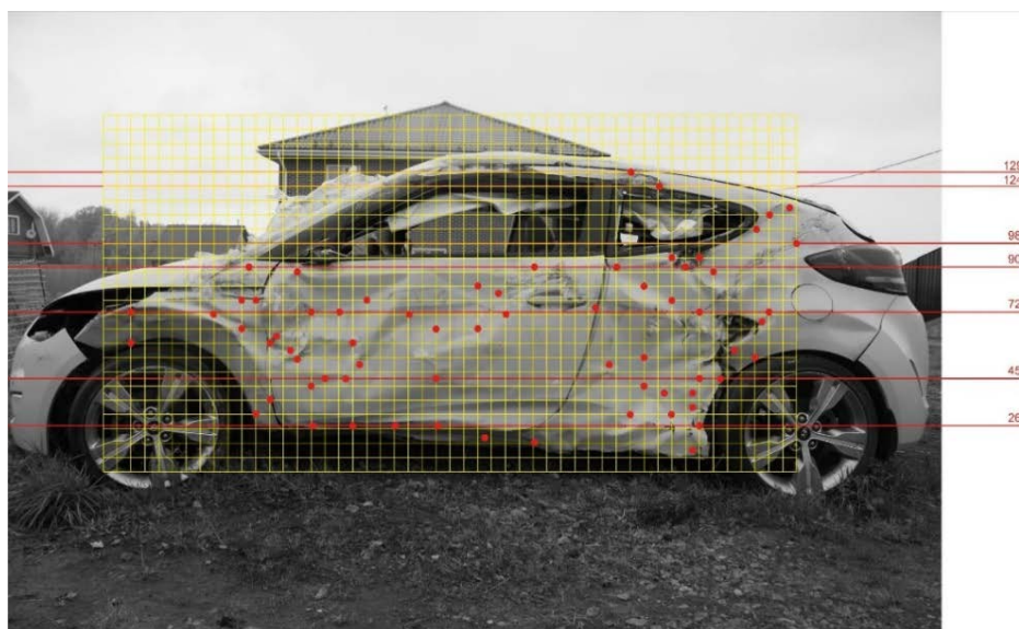
Рисунок 2.24 – Экспликация точек замера от вертикальной плоскости
