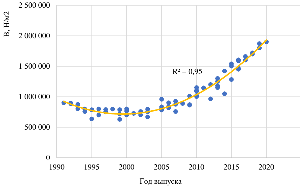
Рисунок 2.19 – Изменение значений модуля упругости I рода фронтальной части кузова автомобиля класса Small MPV в зависимости от года выпуска
