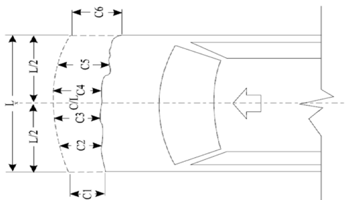
Рисунок 2.2 – Линейная съемка глубины зон деформаций и привязка размеров при фронтальном ударе
