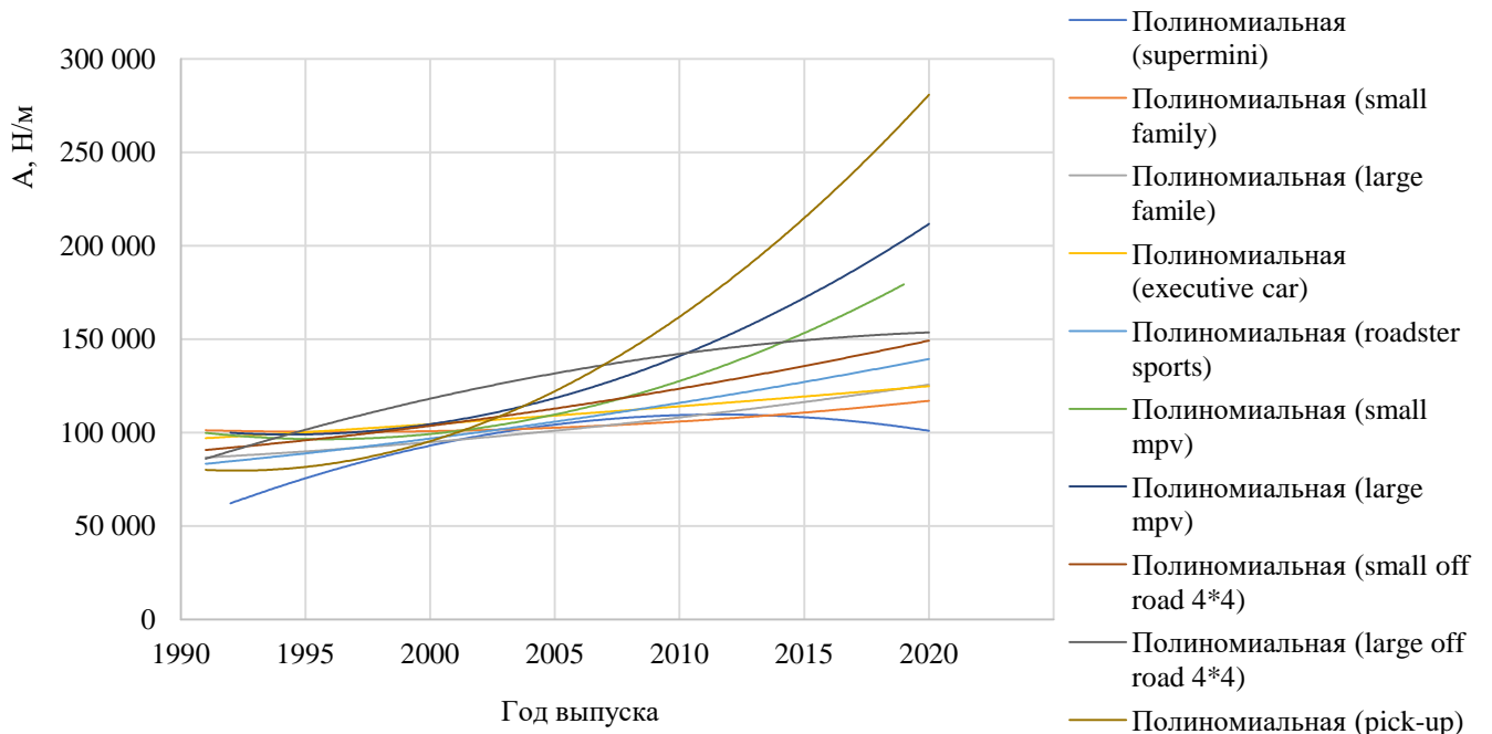
Рисунок П.Б.41 – График изменения значений коэффициента Гука фронтальной части кузова автомобилей разных классов в зависимости от года выпуска
