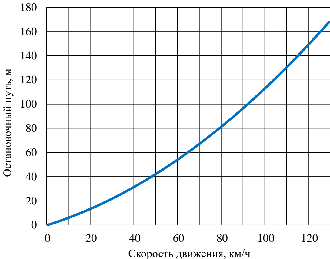
Рисунок 1.2 – График зависимости остановочного пути автомобиля от его скорости движения
