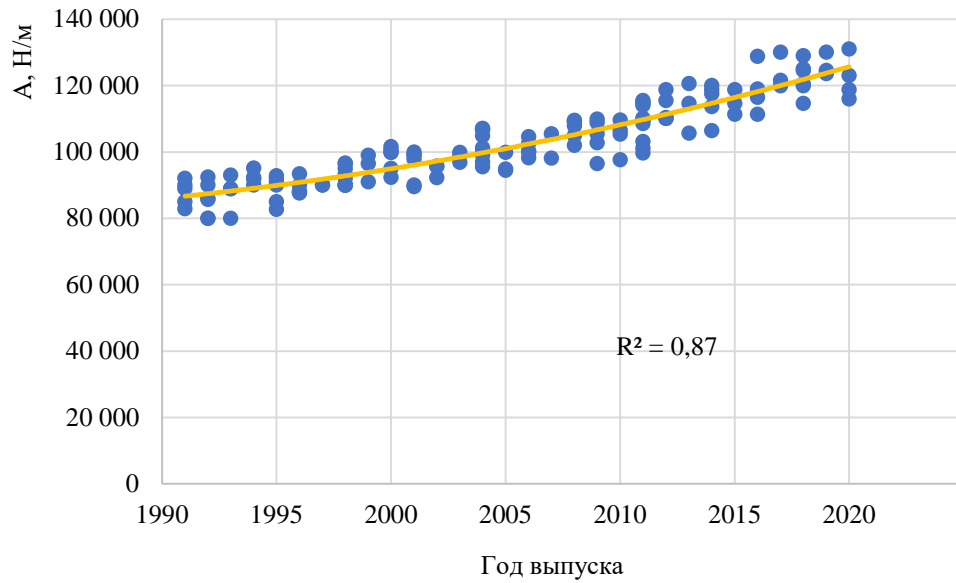
Рисунок П.Б.9 – Изменение значений коэффициента Гука фронтальной части кузова автомобилей класса Large family car в зависимости от года выпуска
