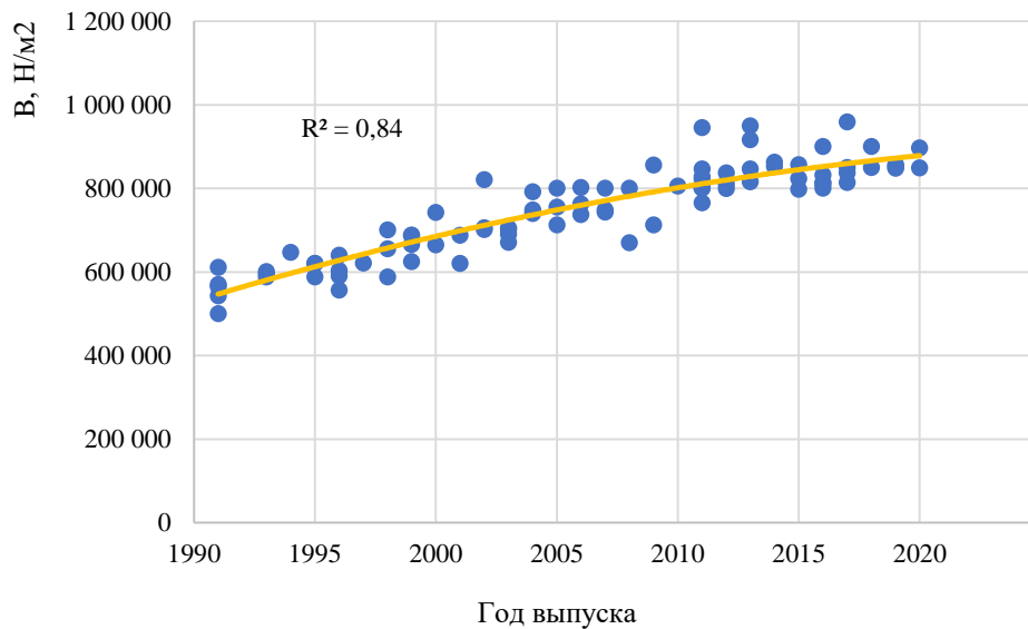
Рисунок П.Б.6 – Изменение значений модуля упругости I рода фронтальной части кузова автомобилей класса Small family car в зависимости от года выпуска
