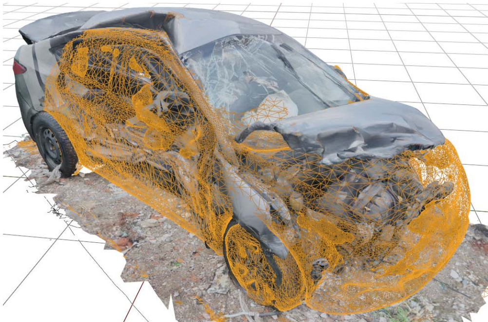
Рисунок 3.33 – Сопоставление 3D-моделей поврежденного и недеформированного состояний автомобиля Hyundai Solaris для производства измерений объемных деформаций
