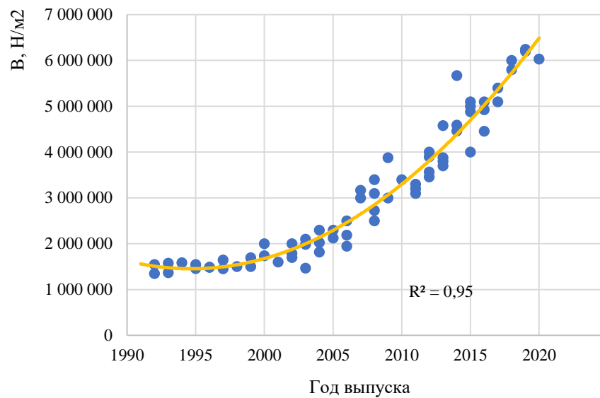
Рисунок П.Б.4 – Изменение значений модуля упругости I рода боковой части кузова автомобилей класса Supermini в зависимости от года выпуска
