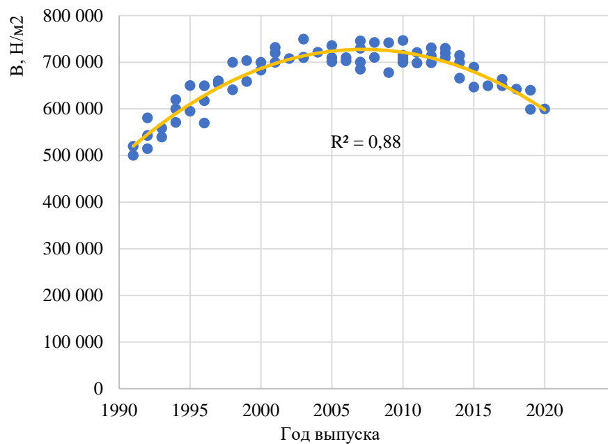
Рисунок П.Б.18 – Изменение значений модуля упругости I рода фронтальной части кузова автомобилей класса Roadster sports в зависимости от года выпуска
