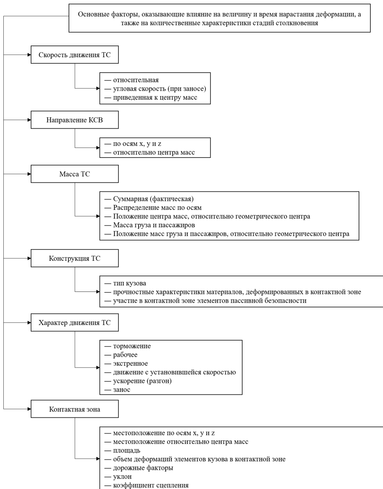
Рисунок 1.8 – Основные факторы, оказывающие влияние на величину и время нарастания деформации, а также на количественные характеристики стадий столкновения ТС
