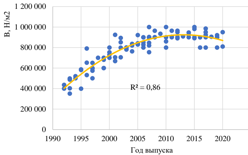
Рисунок П.Б.2 – Изменение значений модуля упругости I рода фронтальной части кузова автомобилей класса Supermini в зависимости от года выпуска
