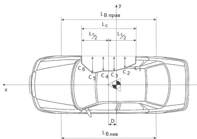
Рисунок 2.1 – Линейная съемка глубины зон деформаций и привязка размеров при боковом ударе
