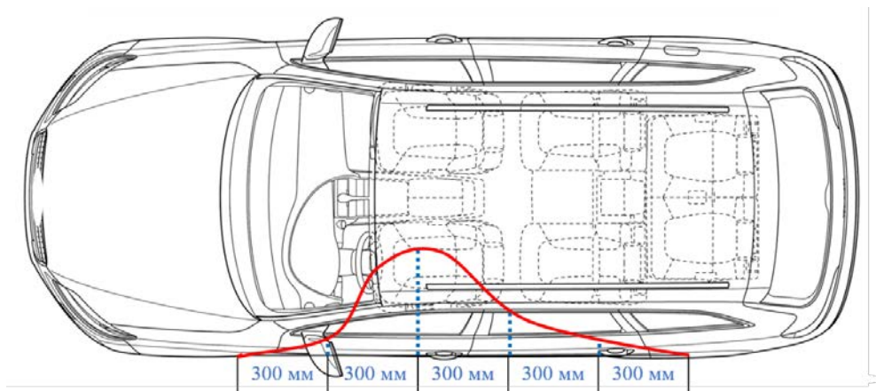
Рисунок 2.15 – Схема участков измерения глубин внедрения с равным шагом
