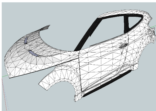
Рисунок 2.25 – 3D-модель кузовных элементов прямой контактной зоны а/м Hyundai Veloster в недеформированном состоянии (вид слева)
