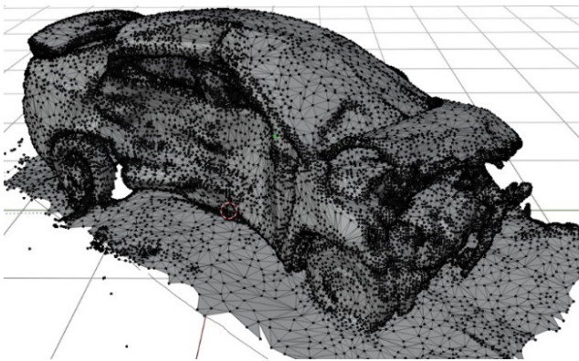
Рисунок 3.30 – 3D-модель деформированного состояния автомобиля Hyundai Solaris, преобразованная в облако точек
