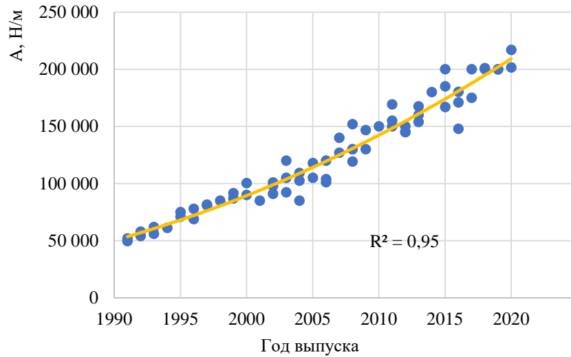
Рисунок П.Б.3 – Изменение значений коэффициента Гука боковой части кузова автомобилей класса Supermini в зависимости от года выпуска
