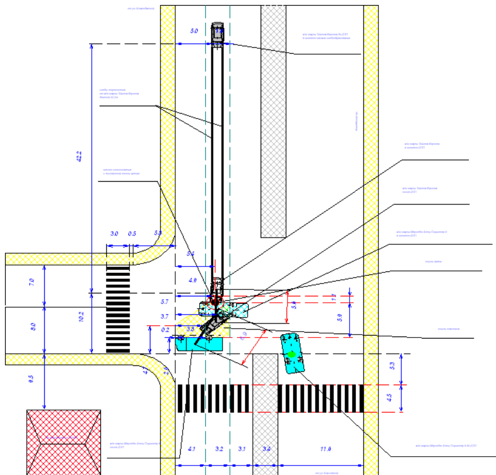
Рисунок 3.11 – Масштабная расчетная схема ДТП с участием а/м Mercedes-Benz Sprinter и а/м Toyota Corolla после ДТП
