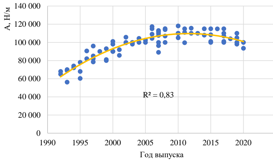
Рисунок П.Б.1 – Изменение значений коэффициента Гука фронтальной части кузова автомобилей класса Supermini в зависимости от года выпуска автомобиля
