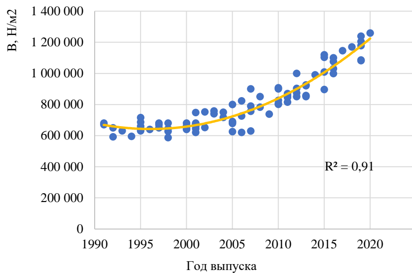
Рисунок П.Б.14 – Изменение значений модуля упругости I рода фронтальной части кузова автомобилей класса Executive car в зависимости от года выпуска
