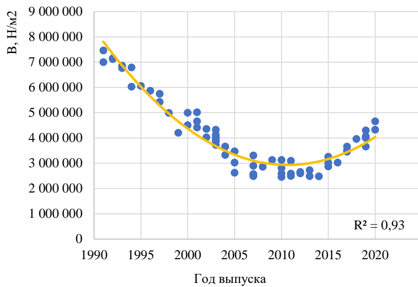
Рисунок П.Б.40 – Изменение значений модуля упругости I рода боковой части кузова автомобилей класса Pick-up в зависимости от года выпуска
