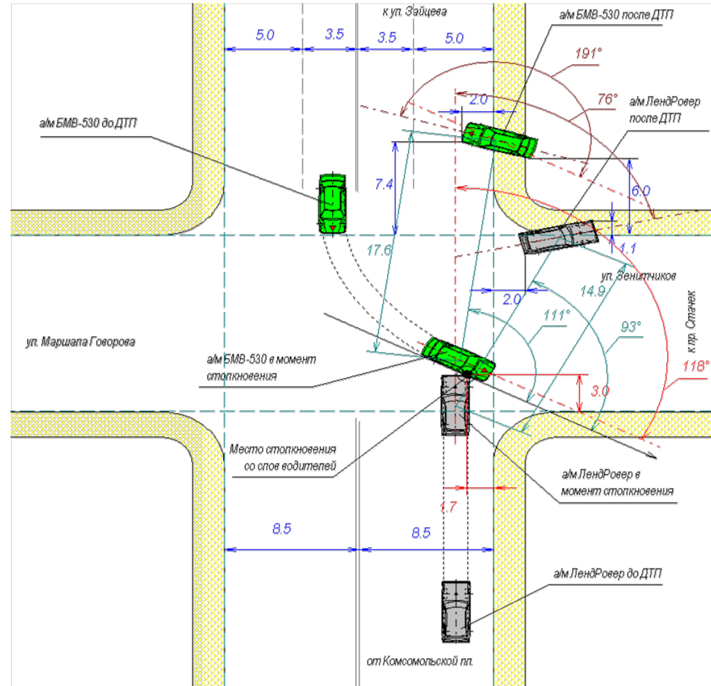
Рисунок 3.23 – Масштабная расчетная схема ДТП с участием а/м BMW 530 и Land Rover Discovery 4
