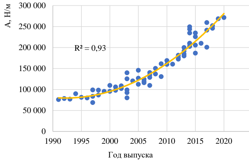
Рисунок П.Б.37 – Изменение значений коэффициента Гука фронтальной части кузова автомобилей класса Pick-up в зависимости от года выпуска
