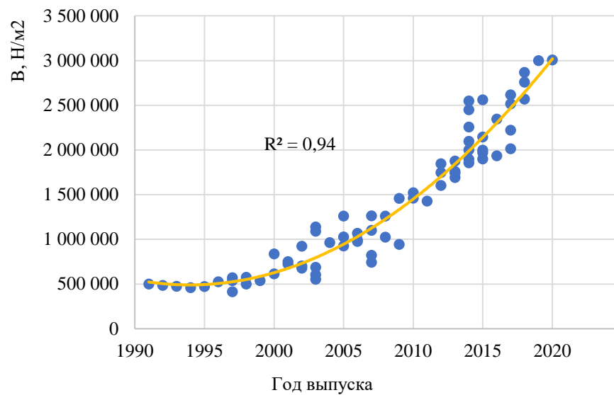
Рисунок П.Б.38 – Изменение значений модуля упругости I рода фронтальной части кузова автомобилей класса Pick-up в зависимости от года выпуска
