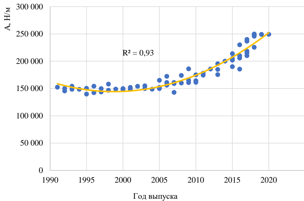
Рисунок 2.20 – Изменение значений коэффициента Гука боковой части кузова автомобиля класса Small MPV в зависимости от года выпуска
