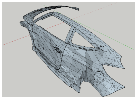
Рисунок 2.28 – 3D-модель кузовных элементов прямой контактной зоны а/м Hyundai Veloster, в деформированном состоянии (вид справа)
