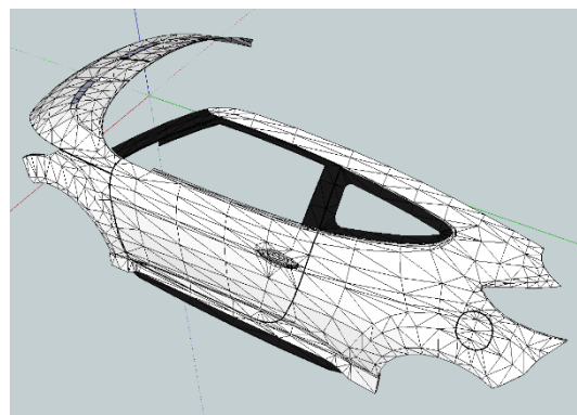
Рисунок 2.26 – 3D-модели кузовных элементов прямой контактной зоны а/м Hyundai Veloster в недеформированном состоянии (вид справа)
