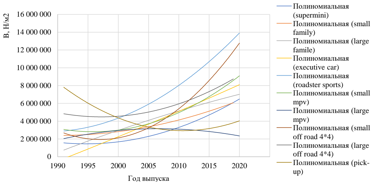
Рисунок П.Б.44 – График изменения значений модуля упругости I рода боковой части кузова автомобилей разных классов в зависимости от года выпуска
