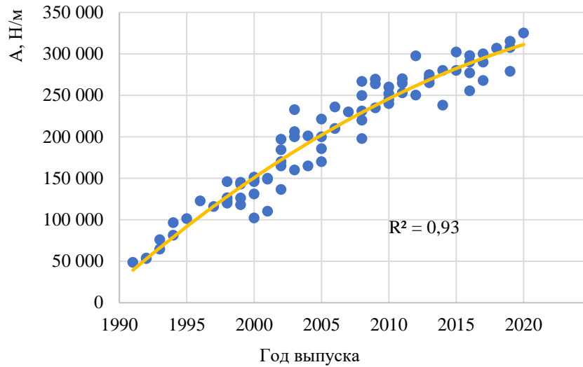
Рисунок П.Б.15 – Изменение значений коэффициента Гука боковой части кузова автомобилей класса Executive car в зависимости от года выпуска
