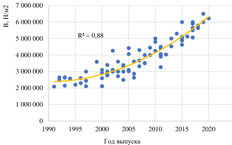
Рисунок П.Б.8 – Изменение значений модуля упругости I рода боковой части кузова автомобилей класса Small family car в зависимости от года выпуска
