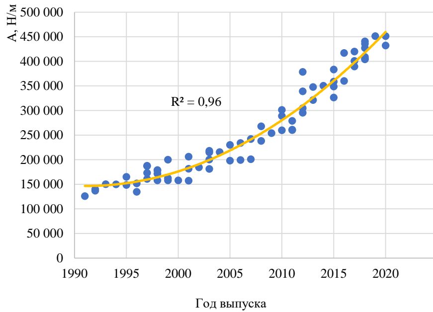
Рисунок П.Б.19 – Изменение значений коэффициента Гука боковой части кузова автомобилей класса Roadster sports в зависимости от года выпуска
