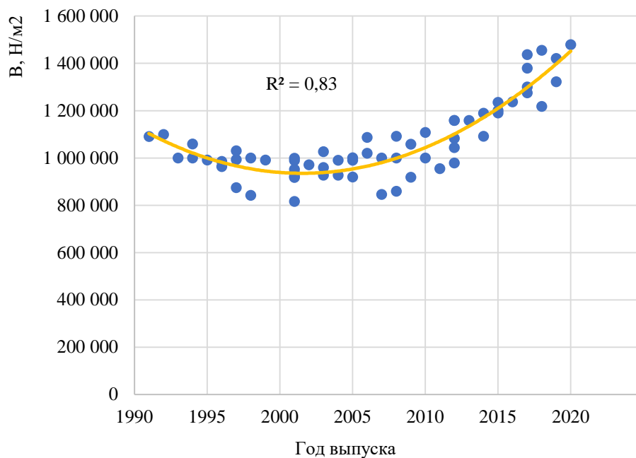
Рисунок П.Б.30 – Изменение значений модуля упругости I рода фронтальной части кузова автомобилей класса Small Off-Road 4×4 в зависимости от года выпуска
