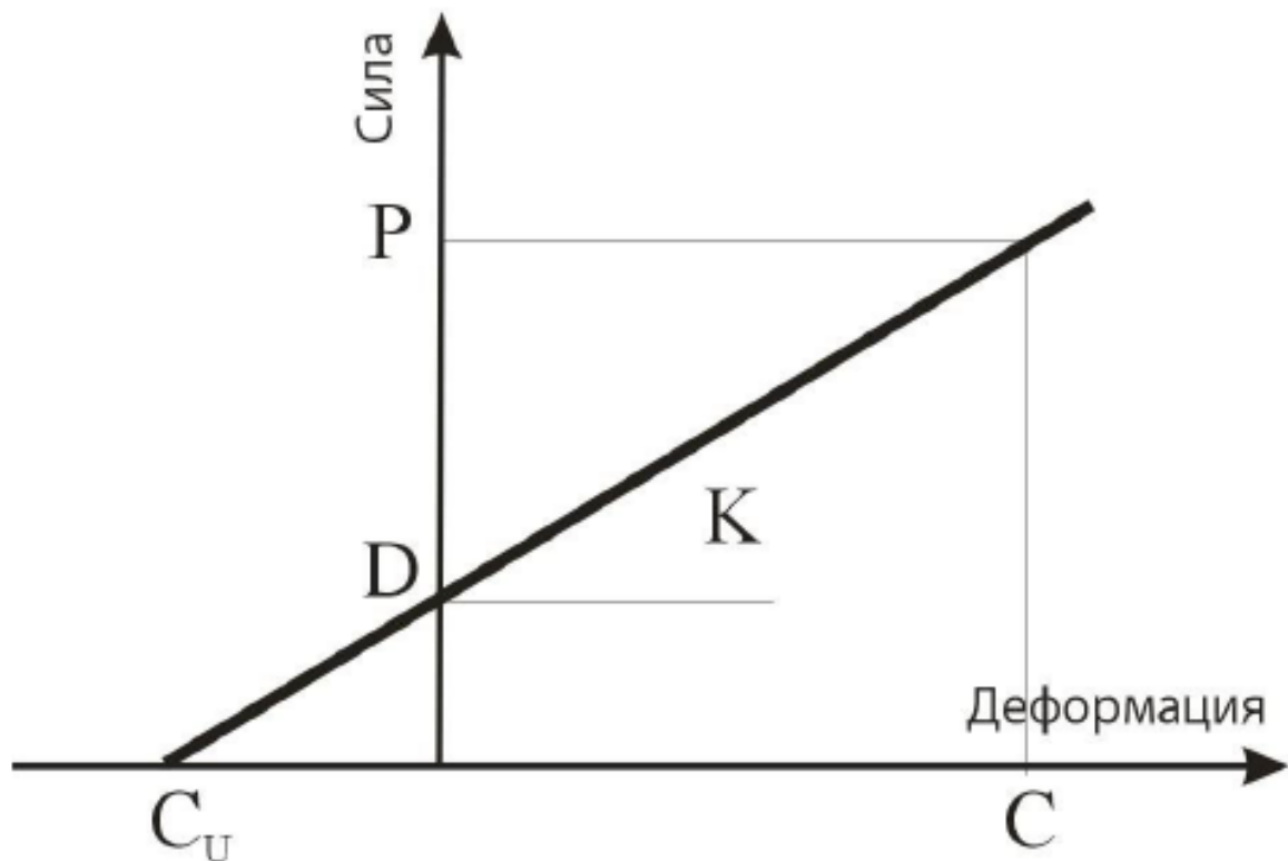
Рисунок 2.3 – График зависимости силы от деформации
