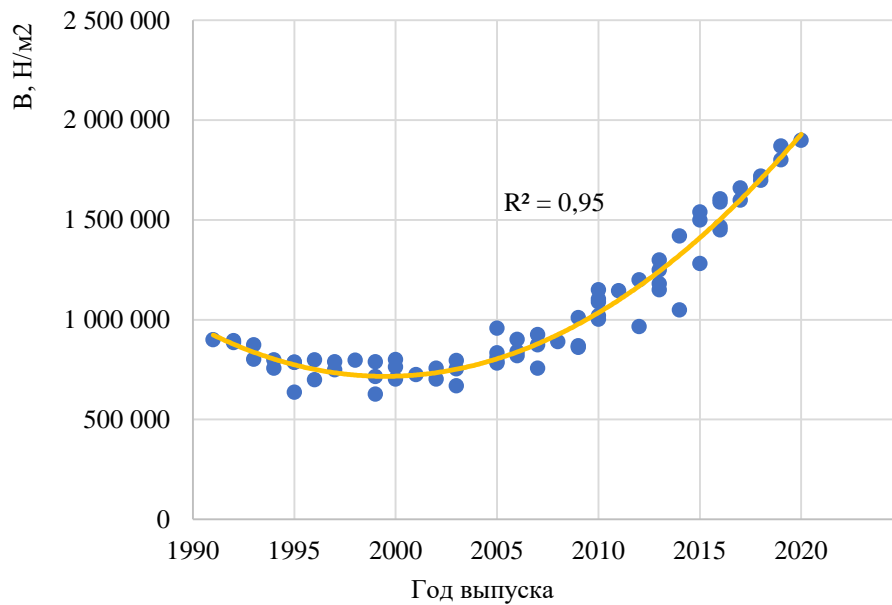
Рисунок П.Б.22 – Изменение значений модуля упругости I рода фронтальной части кузова автомобилей класса Small MPV в зависимости от года выпуска
