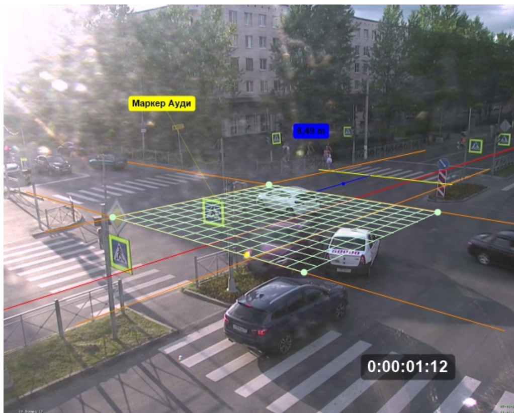
Рисунок 3.7 – Окончание трекинга маркера (положение маркера на Границе 3) и замера времени перемещения
