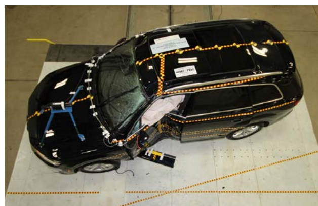
Рисунок 2.14 – Автомобиль Audi Q7 после КСВ с сконцентрированной деформирующей силой
