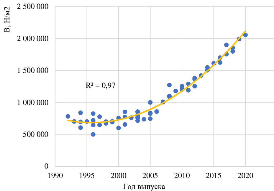
Рисунок П.Б.26 – Изменение значений модуля упругости I рода фронтальной части кузова автомобилей класса Large MPV в зависимости от года выпуска
