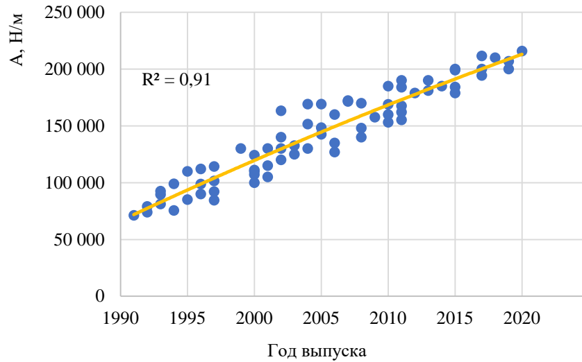
Рисунок П.Б.7 – Изменение значений коэффициента Гука боковой части кузова автомобилей класса Small family car в зависимости от года выпуска
