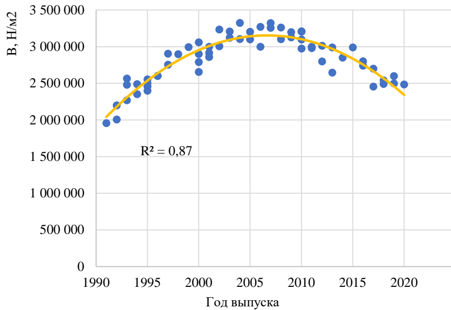
Рисунок П.Б.28 – Изменение значений модуля упругости I рода боковой части кузова автомобилей класса Large MPV в зависимости от года выпуска
