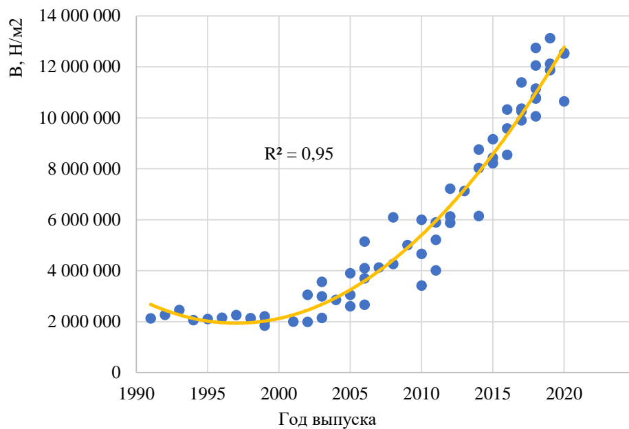
Рисунок П.Б.32 – Изменение значений модуля упругости I рода боковой части кузова автомобилей класса Small Off-Road 4×4 в зависимости от года выпуска
