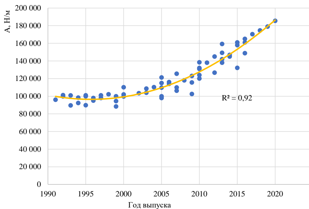
Рисунок 2.18 – Изменение значений коэффициента Гука фронтальной части кузова автомобиля класса Small MPV в зависимости от года выпуска
