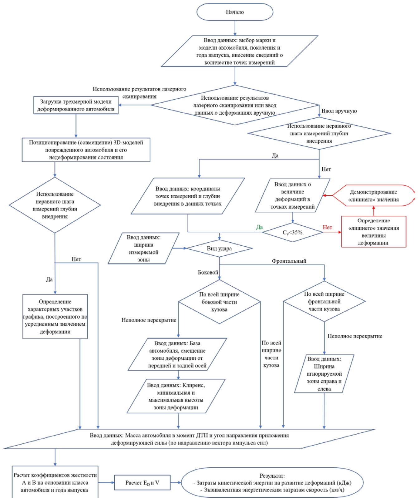
Рисунок 4.2 – Алгоритм расчета скорости автомобиля-участника ДТП в момент столкновения с учётом полученных деформаций
