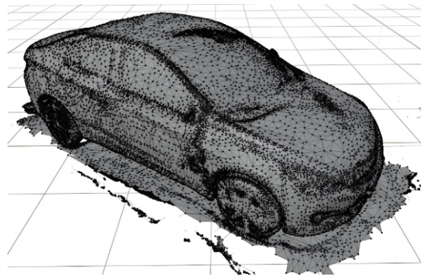
Рисунок 3.31 – 3D-модель исходного (недеформированного) состояния автомобиля Hyundai Solaris в виде облака точек
