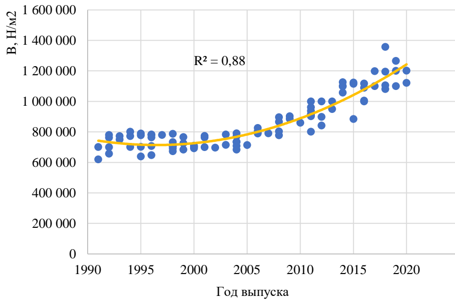
Рисунок П.Б.10 – Изменение значений модуля упругости I рода фронтальной части кузова автомобилей класса Large family car в зависимости от года выпуска
