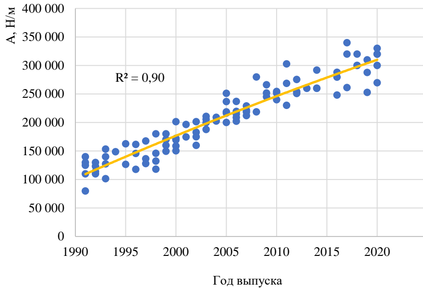
Рисунок П.Б.11 – Изменение значений коэффициента Гука боковой части кузова автомобилей класса Large family car в зависимости от года выпуска
