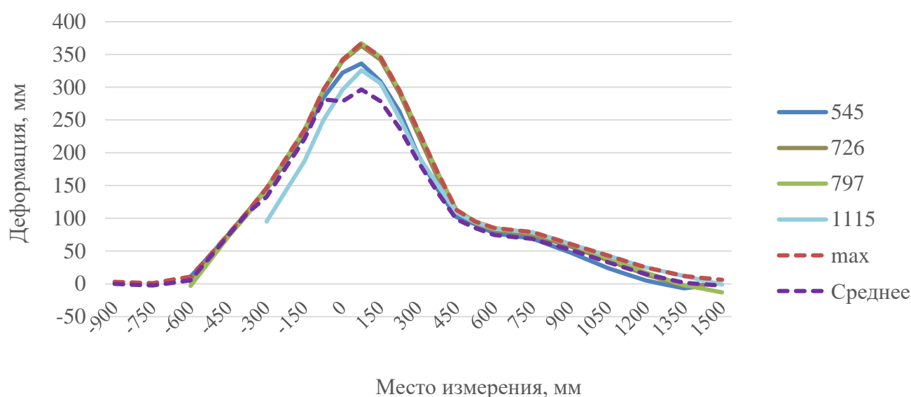
Рисунок 2.16 – График деформации автомобиля Audi Q7 при концентрированном ударе
