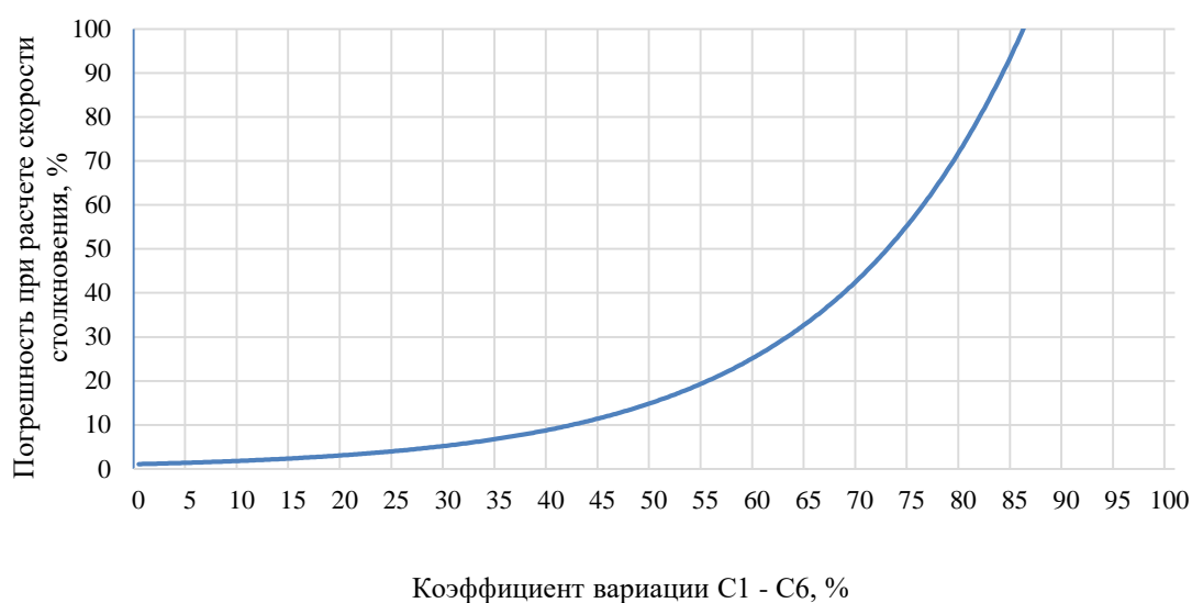
Рисунок 2.10 – Влияние коэффициента вариации измерений глубин внедрений на результаты расчета скорости автомобиля в момент ДТП
