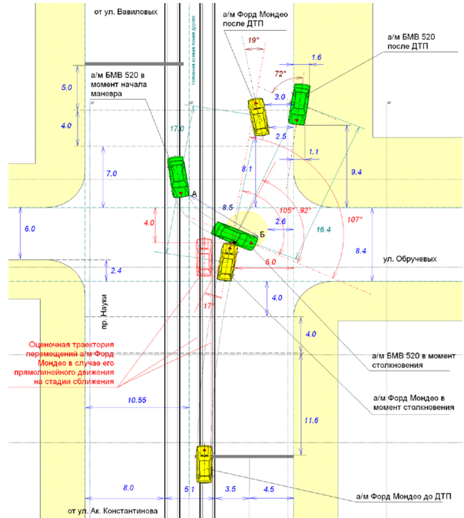
Рисунок 3.13 – А/м BMW 520 в результате ДТП
