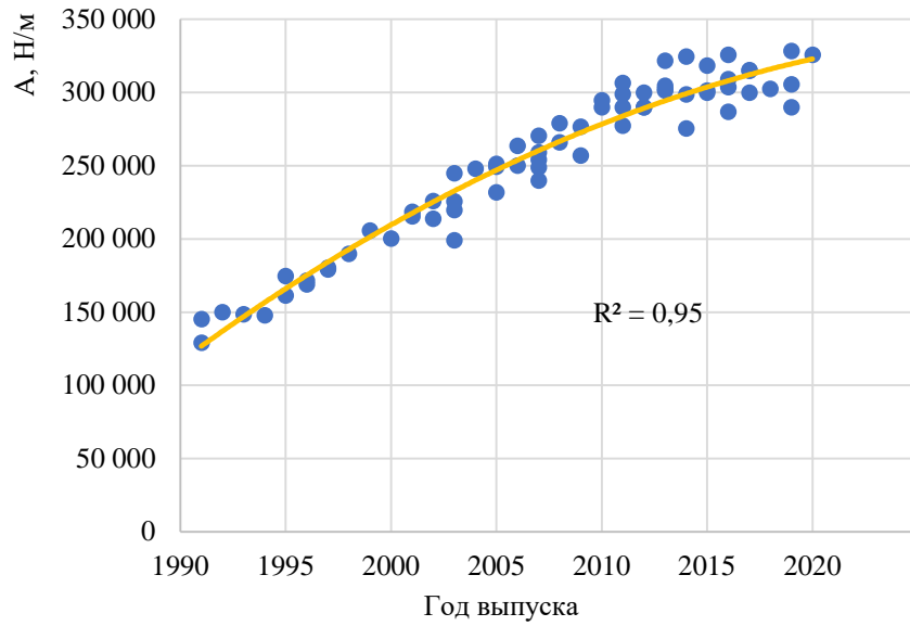
Рисунок П.Б.35 – Изменение значений коэффициента Гука боковой части кузова автомобилей класса Large Off-Road 4×4 в зависимости от года выпуска
