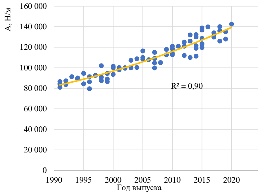
Рисунок П.Б.17 – Изменение значений коэффициента Гука фронтальной части кузова автомобилей класса Roadster sports в зависимости от года выпуска
