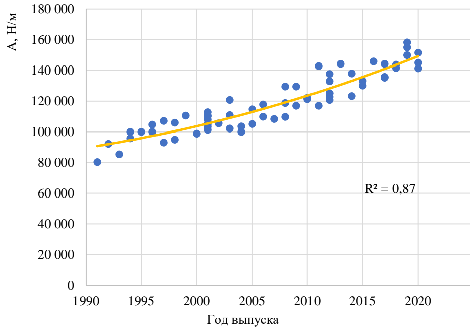
Рисунок П.Б.29 – Изменение значений коэффициента Гука фронтальной части кузова автомобилей класса Small Off-Road 4×4 в зависимости от года выпуска
