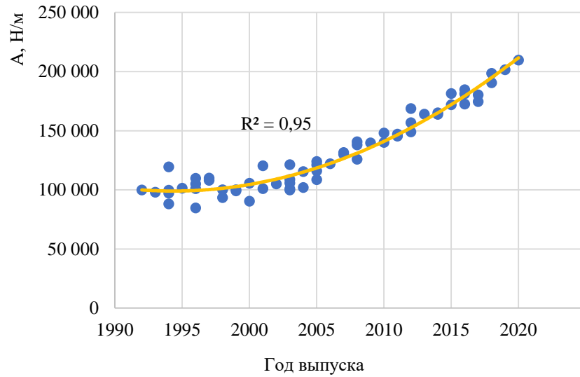
Рисунок П.Б.25 – Изменение значений коэффициента Гука фронтальной части кузова автомобилей класса Large MPV в зависимости от года выпуска
