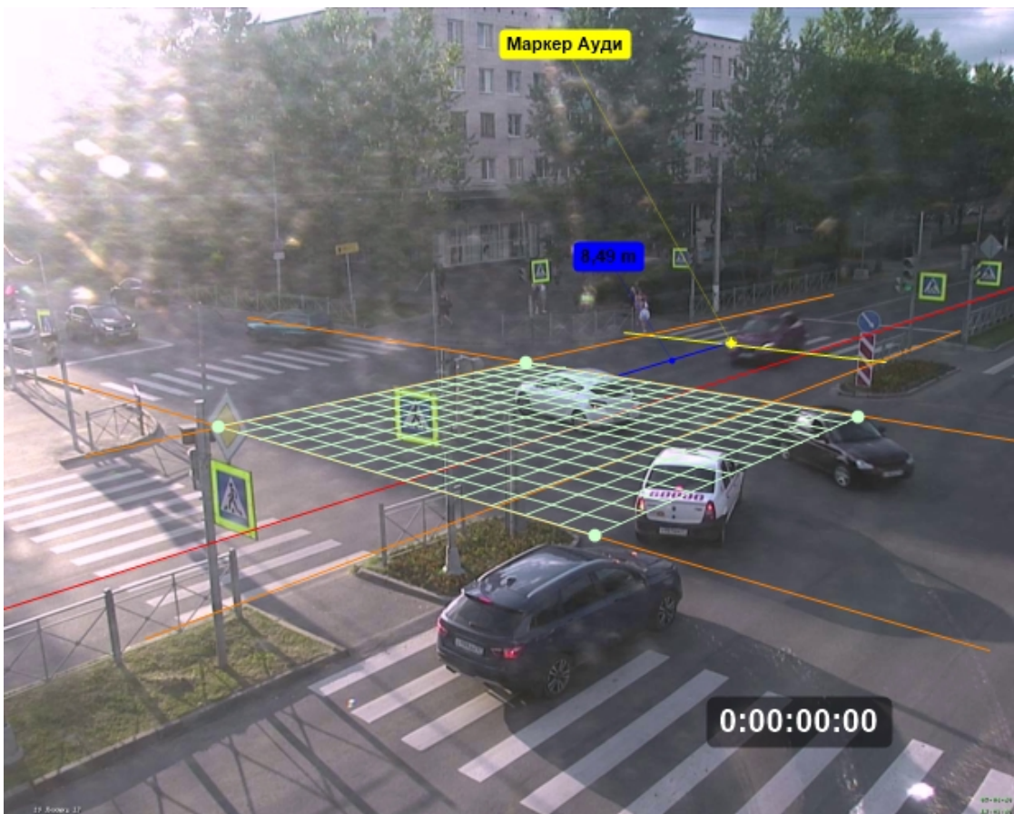
Рисунок 3.5 – Начало трекинга маркера (положение маркера на Границе 1) и замера времени перемещения
