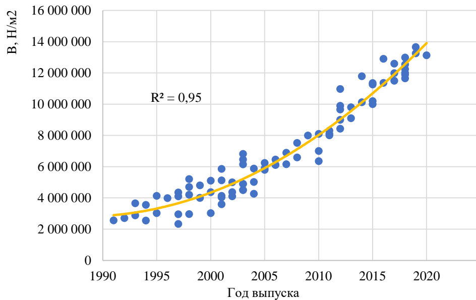
Рисунок П.Б.20 – Изменение значений модуля упругости I рода боковой части кузова автомобилей класса Roadster sports в зависимости от года выпуска
