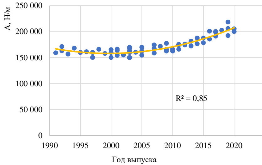
Рисунок П.Б.39 – Изменение значений коэффициента Гука боковой части кузова автомобилей класса Pick-up в зависимости от года выпуска
