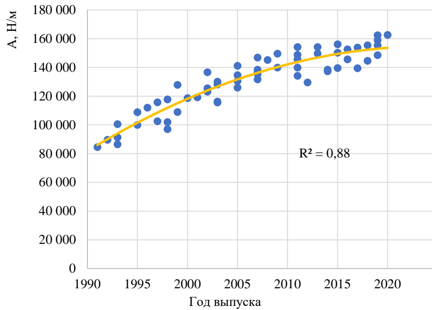
Рисунок П.Б.33 – Изменение значений коэффициента Гука фронтальной части кузова автомобилей класса Large Off-Road 4×4 в зависимости от года выпуска
