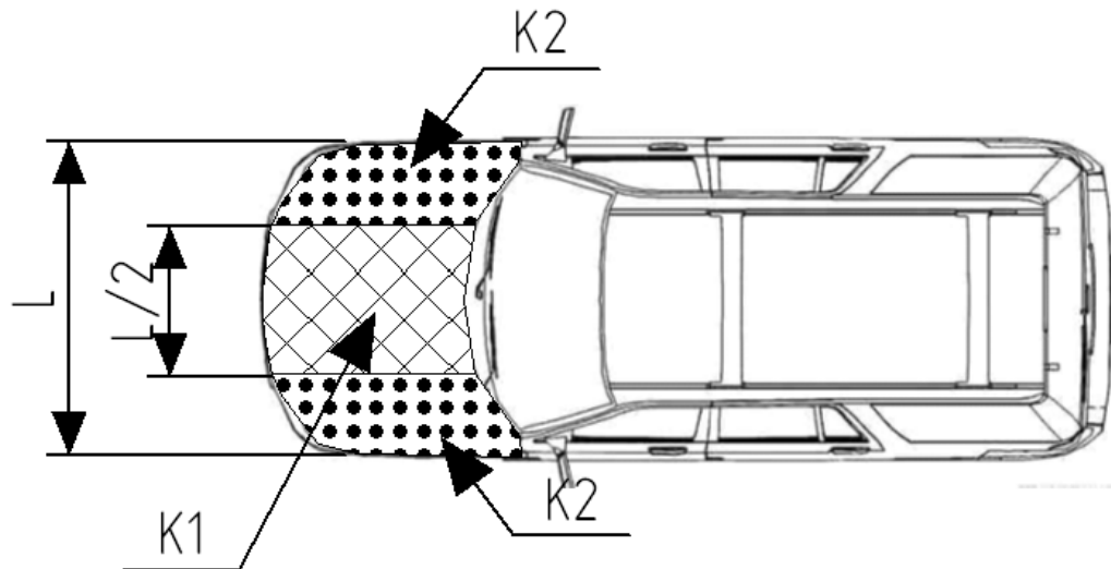
Рисунок 2.4 – Конструкционная жесткость передней части автомобиля
