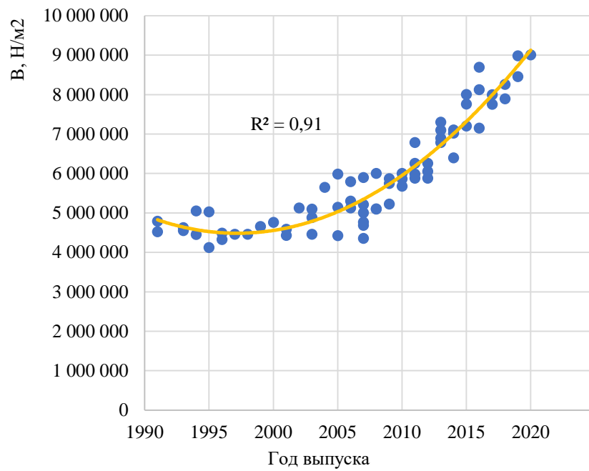
Рисунок П.Б.36 – Изменение значений модуля упругости I рода боковой части кузова автомобилей класса Large Off-Road 4×4 в зависимости от года выпуска
