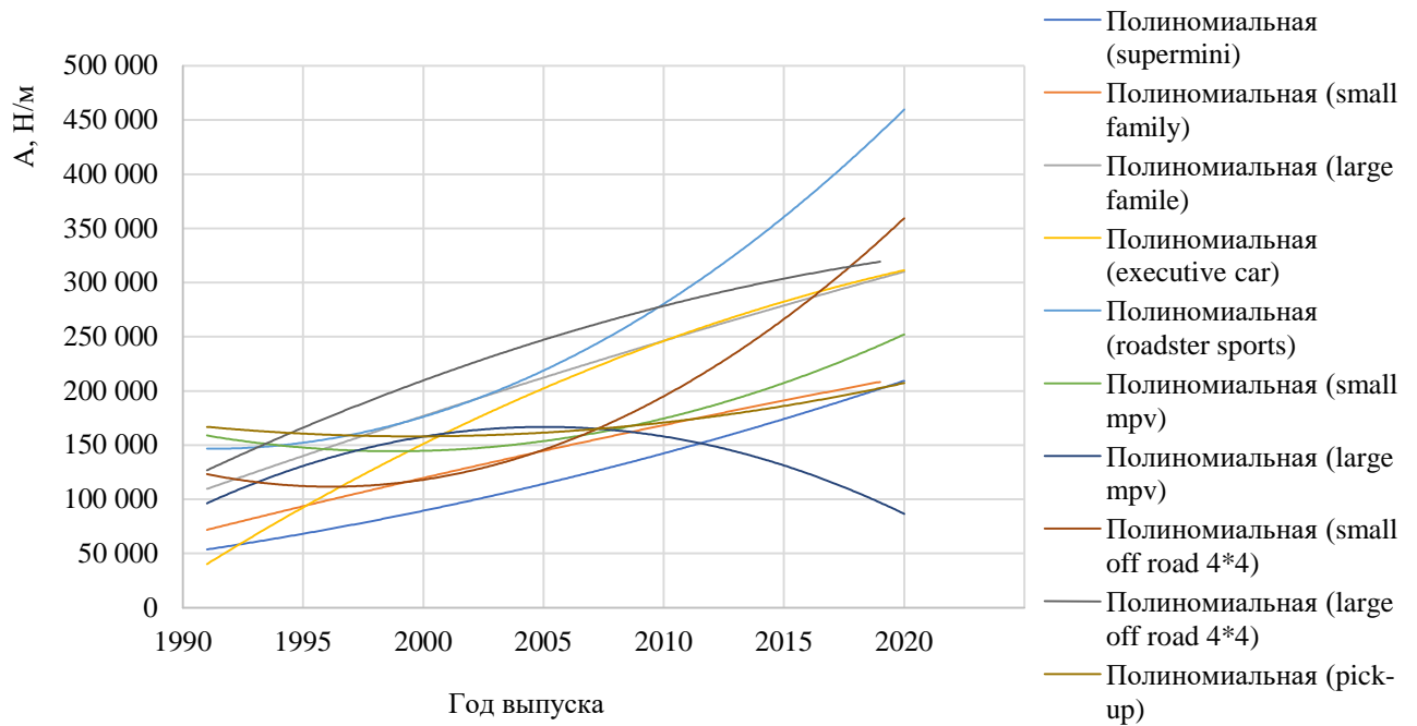
Рисунок П.Б.43 – График изменения значений коэффициента Гука боковой части кузова автомобилей разных классов в зависимости от года выпуска
