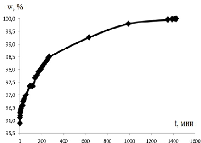
Рис.3. График регидратации сорбента №1
