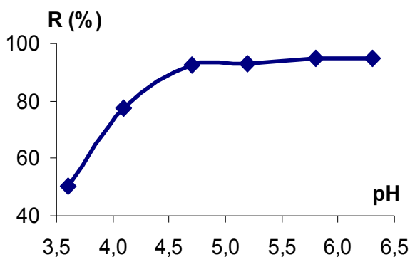
Рис. 1 Оптимальное pH сорбции железа(III) природным цеолитом
