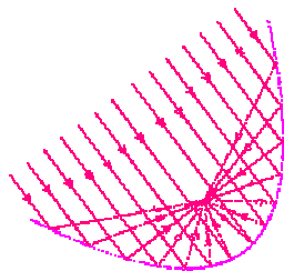
Рис.2. Параллельные лучи поступают слева, и доводится до фокуса к одной точке
