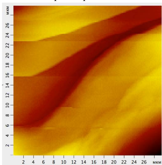
Рис.3 СЗМ-кадр поверхности NaCl.
