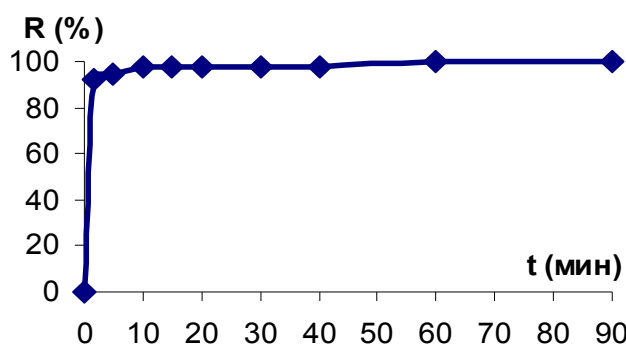
Рис. 4 Оптимальное время сорбции Fe(III) синтетическим цеолитом
