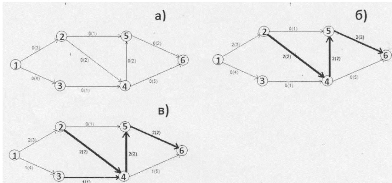
Рис. 1 а) Исходный граф; б) Формирование потока. Итерация I; в) Формирование потока. Итерация II.
