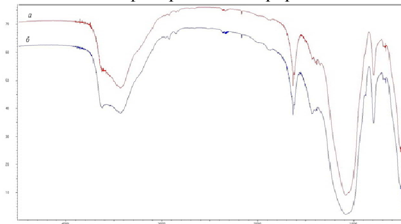
Рис. 1. Инфракрасные спектры поглощения природного(а) и модифицированного(б) цеолитов [спектрометр ФСМ 2202; условия получения: таблетирование 1мг исследуемого вещества с 0,3 г KBr]
