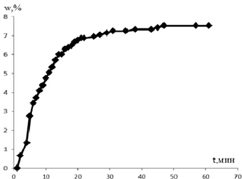
Рис. 2. График дегидратации сорбента №1
