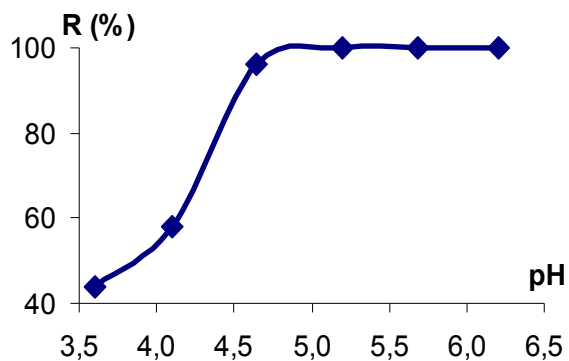
Рис. 2 Оптимальное pH сорбции железа(III) синтетического цеолита
