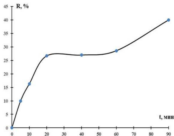
Рис.3. Влияние времени сорбции на степень извлечения 2,4-Д кислоты
