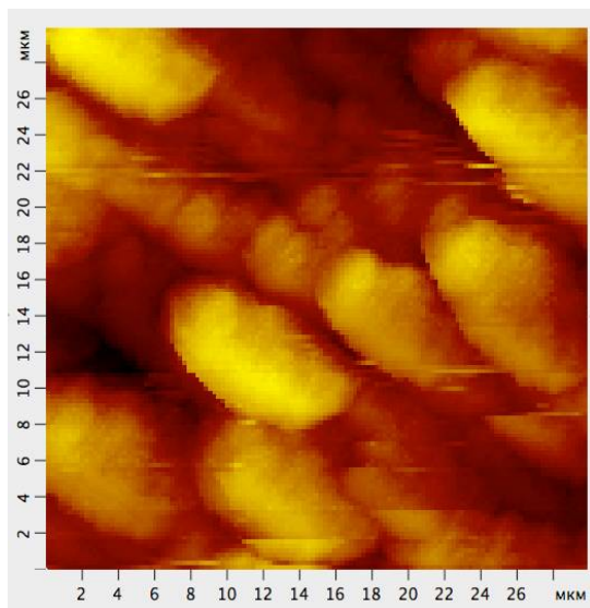
Рис.2 СЗМ-кадр поверхности пленки NaCl.
