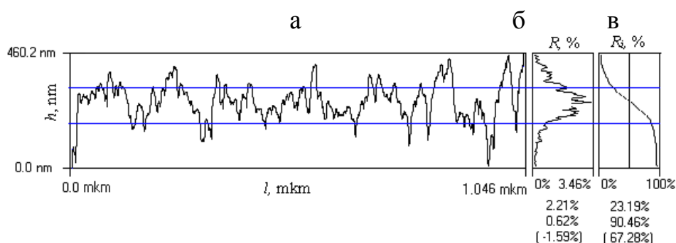
Рис. 2. Интегральный профиль поверхности ПКС (а), гистограмма распределения точек профиля поверхности ПКС по высотам (б) и график интеграла от гистограммы по высотам (в); h, \text{нм} - высота профиля рельефа вдоль скана с размером l, \text{мкм} . R - количество точек профиля (в % от общего количества), имеющих данную высоту и R_i - количество точек профиля (в % от общего количества), имеющих высоту большую или равную данной
