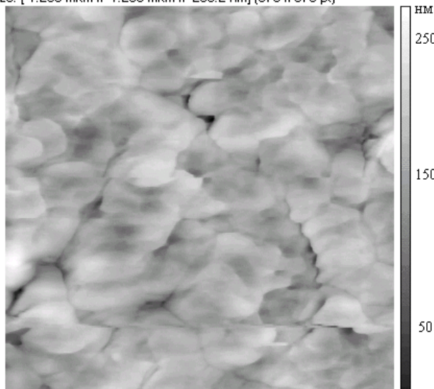
Рис. 3. Поверхность ПКС в виде «пластинок» после нагревания образца в течение 30 минут при температуре 120 \pm 1^\circ\text{C} . Количество точек, формирующих изображение: 673×673
