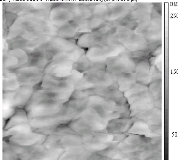
Рис. 3. Поверхность ПКС в виде «пластинок» после нагревания образца в течение 30 минут при температуре 120 \pm 1^\circ\text{C} . Количество точек, формирующих изображение: 673 \times 673
