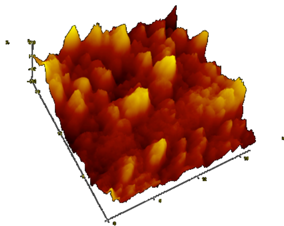
Рис. 2. Типичное 3D АСМ-изображение морфологии поверхности кристалла \text{BaTiO}_3
