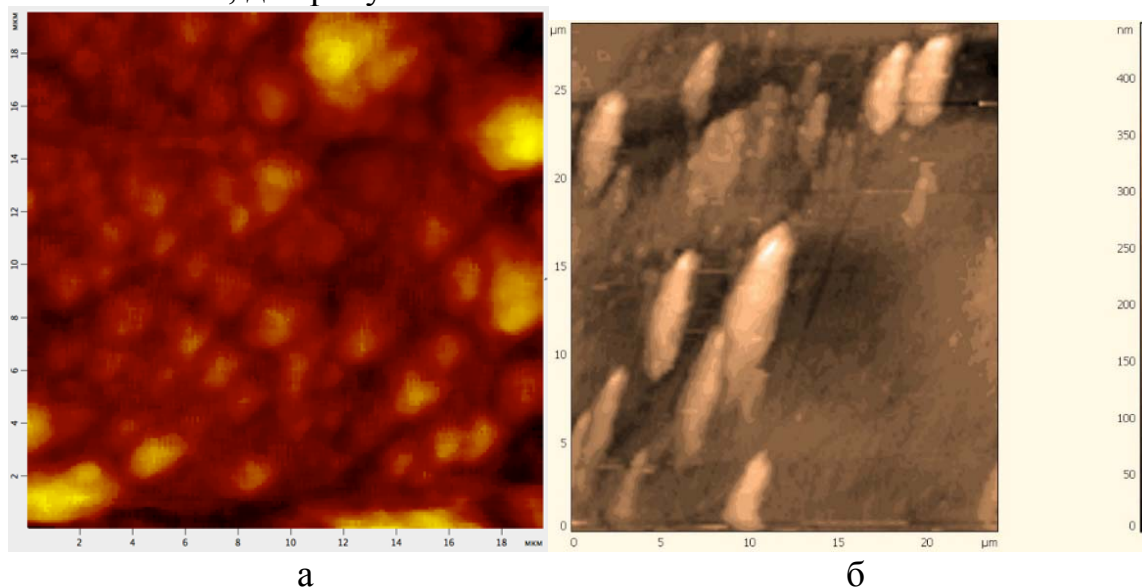
Рис. 1. Типичное АСМ-изображение морфологии поверхности кристалла \text{BaTiO}_3
