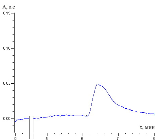
Рис. 3. Хроматограмма стандартного образца доксициклина, [ДЦ] = 4 \cdot 10^{-6} г/мл, \lambda = 350 нм, pH \approx 3.5
