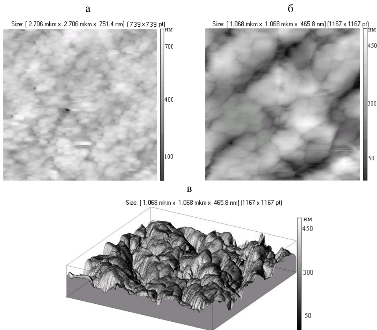
Рис. 1. Типичное АСМ изображение поверхности ПКС в 2D (а, б) и 3D (в) виде.
