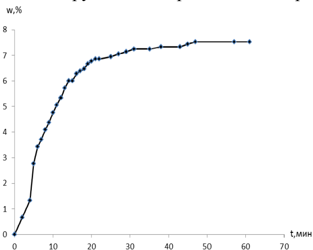
Рис. 2. График дегидратации сорбента №1
