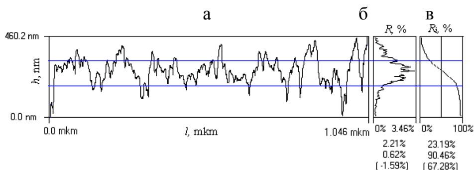
Рис. 2. Интегральный профиль поверхности ПКС (а), гистограмма распределения точек профиля поверхности ПКС по высотам (б) и график интеграла от гистограммы по высотам (в); h, \text{нм} - высота профиля рельефа вдоль скана с размером l, \text{мкм} . R - количество точек профиля (в % от общего количества), имеющих данную высоту и R_i - количество точек профиля (в % от общего количества), имеющих высоту большую или равную данной
