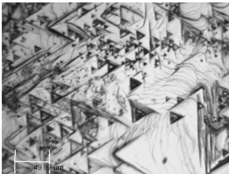
Рис. 1. МГМ – изображение кристалла висмут – сурьма после травления.
