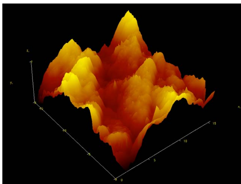
Рис. 2 3D-изображение АСМ-кадра первого участка синтетического кристалла цеолита после вычитания постоянной по Y
