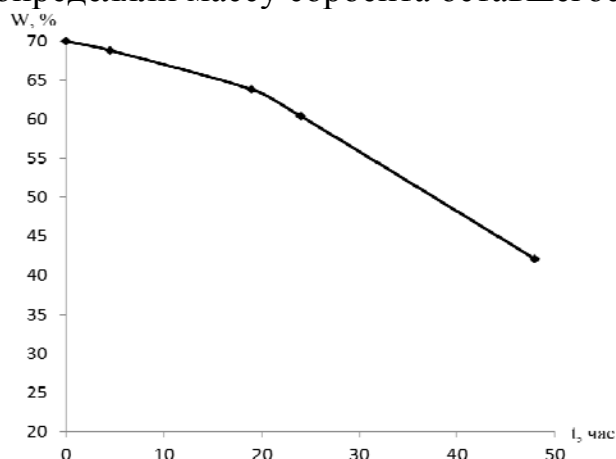
Рис. 1. Изменение массы сорбента №1 на поверхности воды с течением времени
