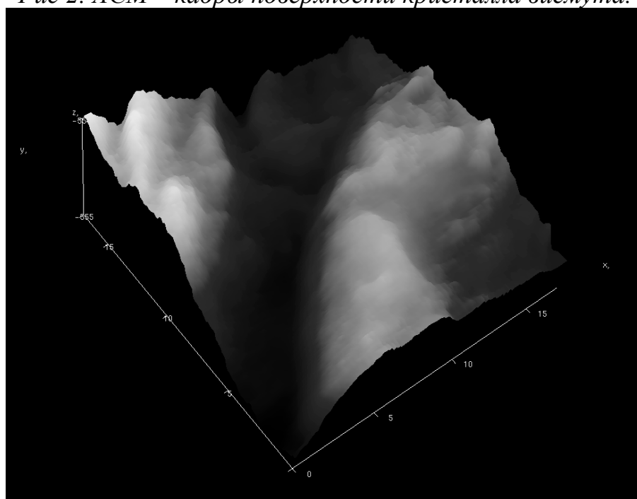
Рис.3.Трехмерное АСМ-изображение участка поверхности скола монокристалла висмута.
