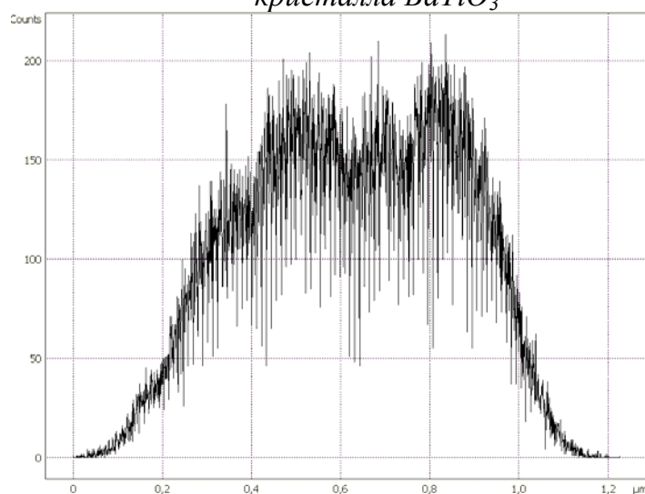
Рис. 3. Типичная гистограмма высот точек поверхности кристалла \text{BaTiO}_3
