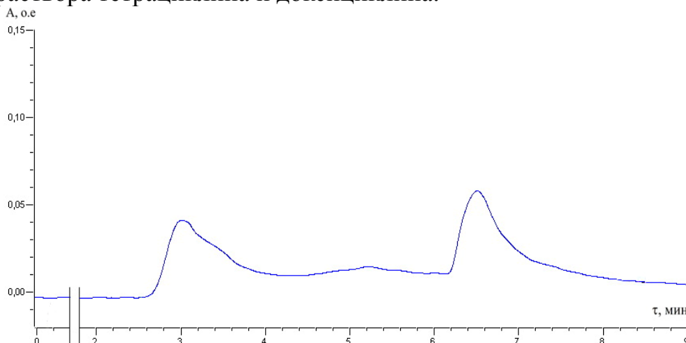
Рис. 4. Хроматограмма модельной смеси тетрациклина и доксициклина; [ТЦ] = 4 \cdot 10^{-6} г/мл, [ДЦ] = 4 \cdot 10^{-6} г/мл, \lambda = 350 нм, pH \approx 3.5
