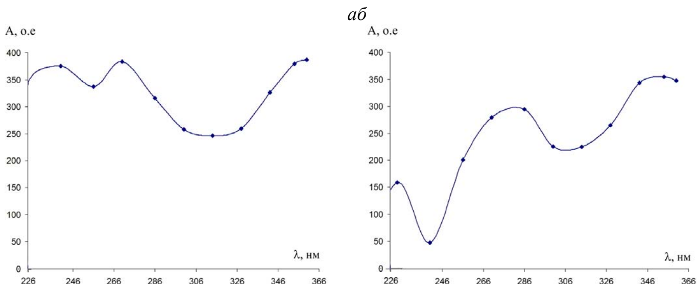
Рис. 1. УФ-спектры модельных растворов ТЦ (а) и ДЦ (б) в воде, pH \approx 6.3
