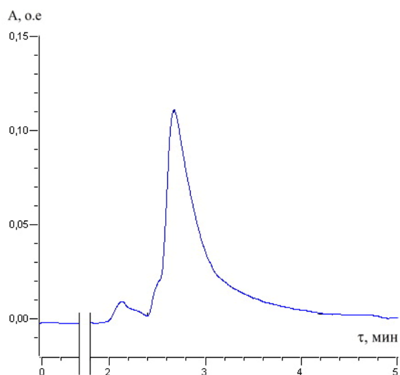
Рис. 2. Хроматограмма стандартного образца тетрациклина, [ТЦ] = 4 \cdot 10^{-6} г/мл, \lambda = 350 нм, pH \approx 3.5
