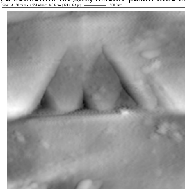
Рис. 3. АСМ-изображение кристалла висмут-сурьмы после травления
