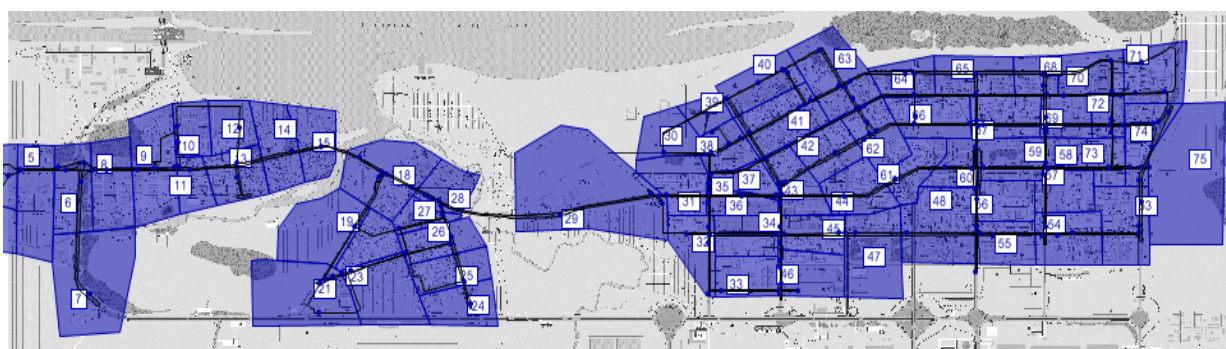
Рисунок 4.3 – Разделение города на транспортные районы
